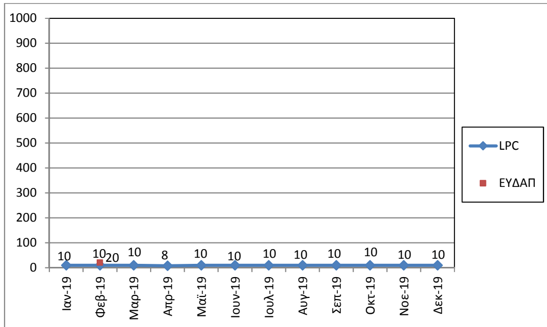
Σχήμα 2-2: Μετρήσεις COD (mg/l) στην εκροή της μονάδας επεξεργασίας υγρών αποβλήτων το 2019, από το εργαστήριο της LPC (μηνιαία μέτρηση) κι από το εργαστήριο της ΕΥΔΑΠ (1 δείγμα για το 2019) σε σύγκριση με το όριο διάθεσης (1000 mg/l)
